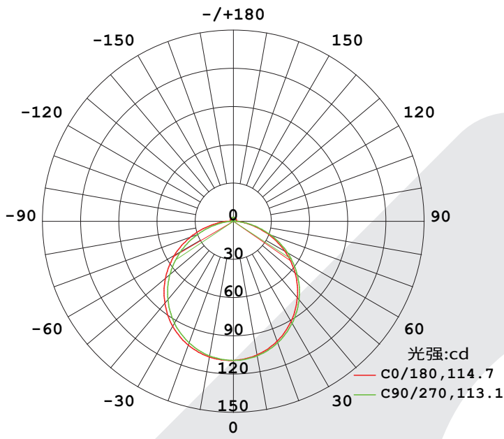
配光曲线
